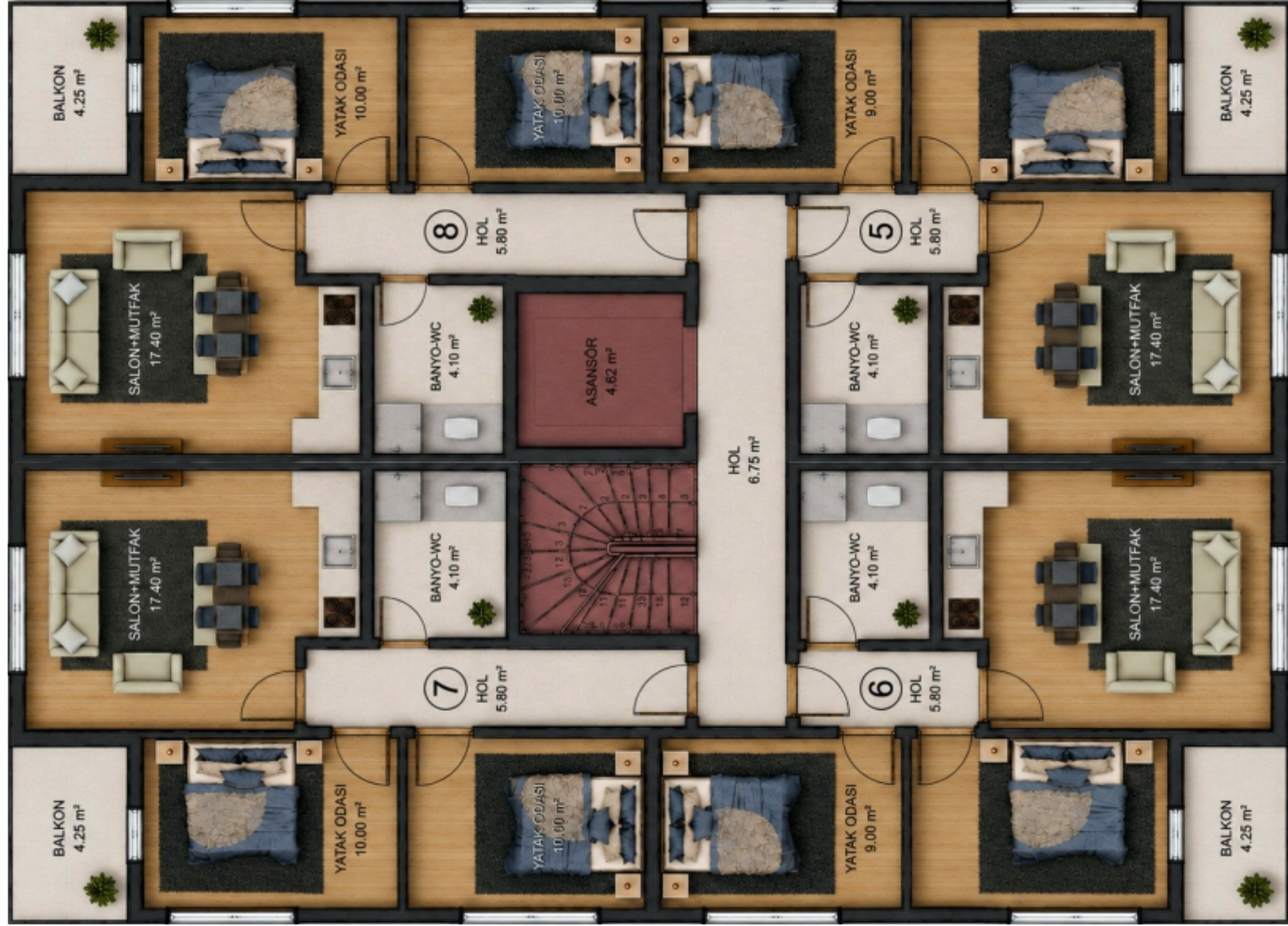
1. KAT PLANI
